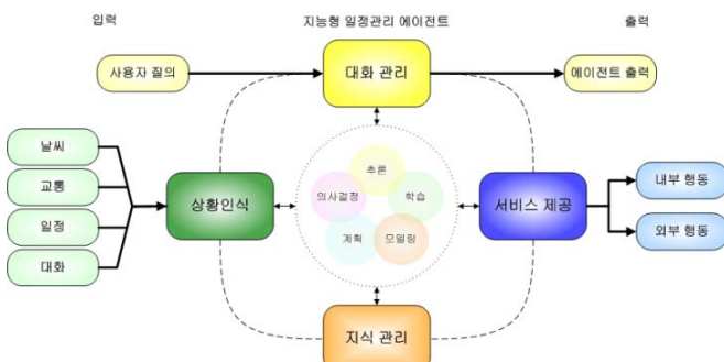
그림 2. 제안하는 지능형 일정관리 에이전트 구조
