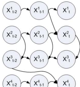
그림 1. 동적 베이지안 네트워크 예
