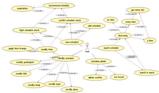
(그림 2) 대화 흐름 Use case
