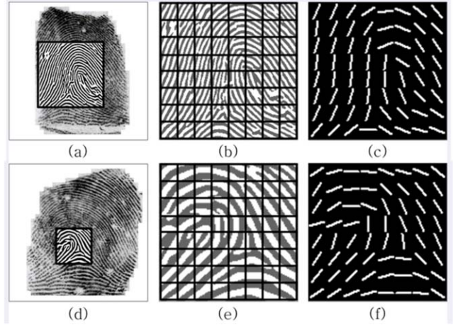
그림 3. 특징영역의 방향성필드. (a) 특징영역의 영상개선, (b) 8 \times 8 개의 블록으로 나눈 특징영역, (c) 특징영역의 방향성필드. (d)~(f)는 다른 지문영상의 예.
