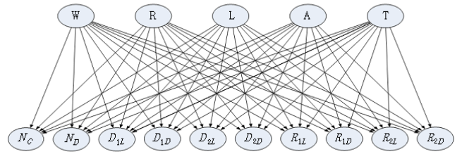
그림 2. 지문분류를 위한 나이브 베이즈 분류기 구조
