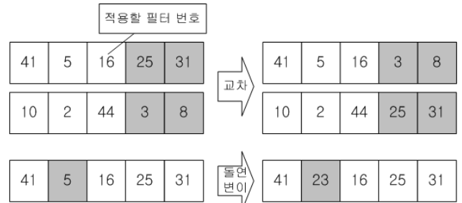
그림 2. 검색체 구조 및 유전자 연산
