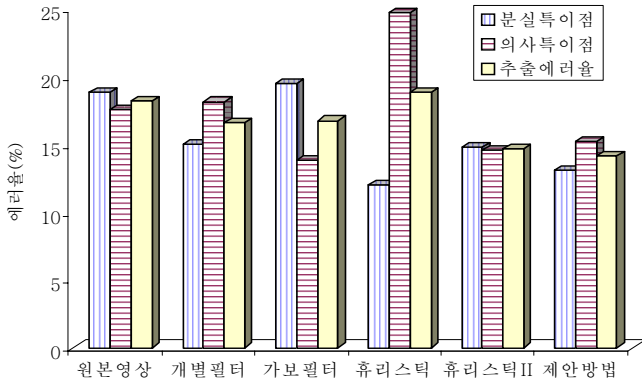
그림 3. 영상필터 성능비교
