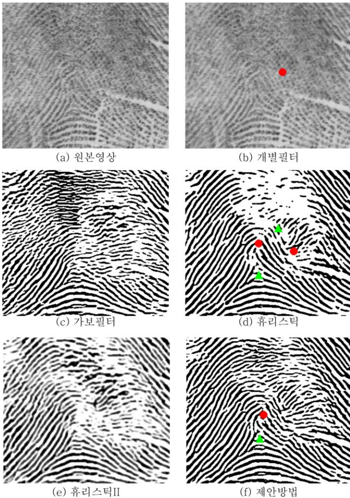
그림 4. 지문영상의 영상필터 효과 (●=중심점, ▲=삼각주)
