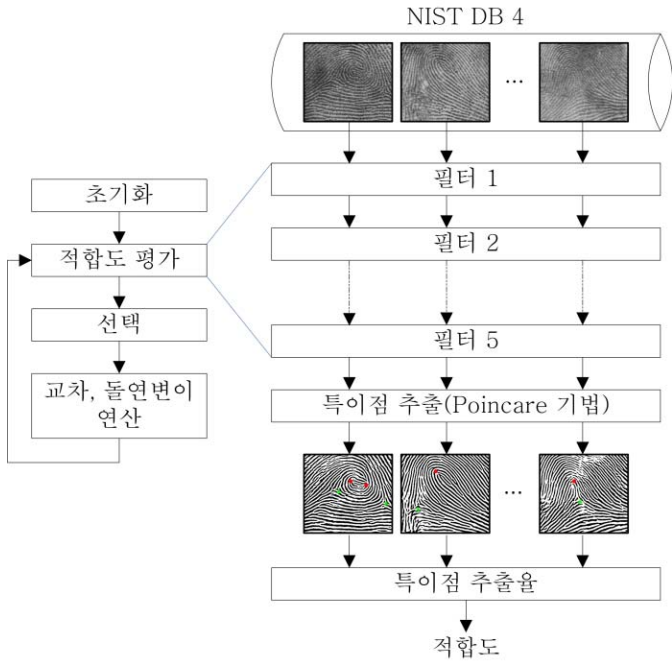
그림 1. 제안하는 방법의 수행과정
