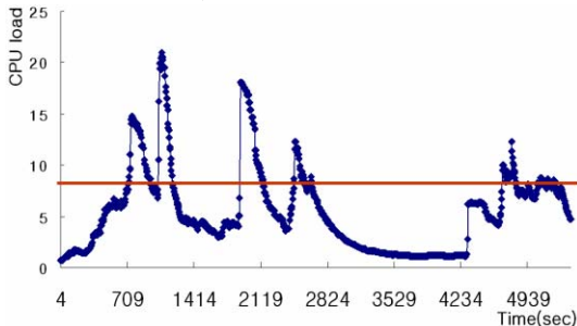
그림 5. cpu상태 그래프
