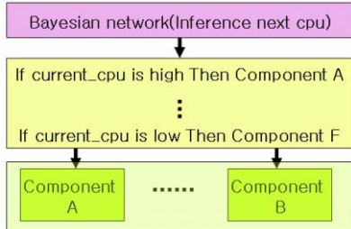
그림 4. if - then 규칙을 이용한 컴포넌트 재구성
