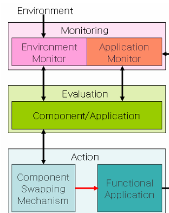
그림 1. 컴포넌트 재구성 가능 미들웨어의 구조
