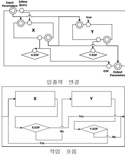
그림 7. X \infty Y (INNER JOIN조합)
