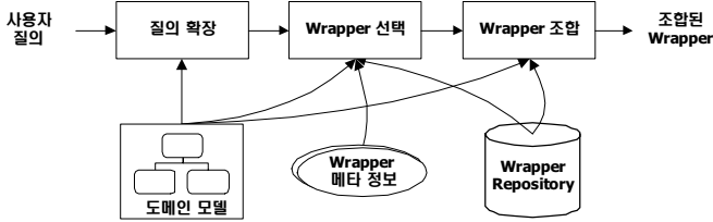
그림 2. 동적 Wrapper 조합과정
