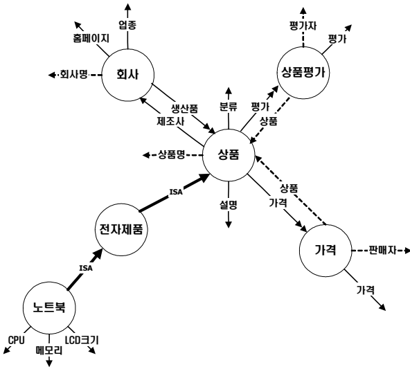
그림 3. 도메인 모델의 예 (온라인 쇼핑분야)
