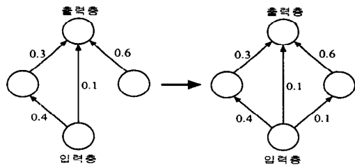
그림 4. 돌연변이 연산
