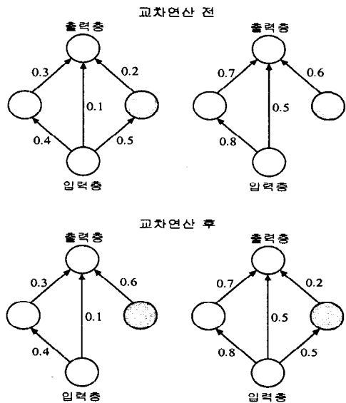
그림 3. 교차 연산
