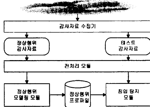
그림 1. 제안하는 탐지방법의 구조
