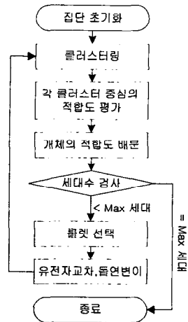
그림 3. 클러스터링 유전자 알고리즘
