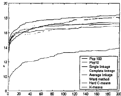
그림 4. De Jong Function 3에 대한 각 알고리즘의 진화 결과
