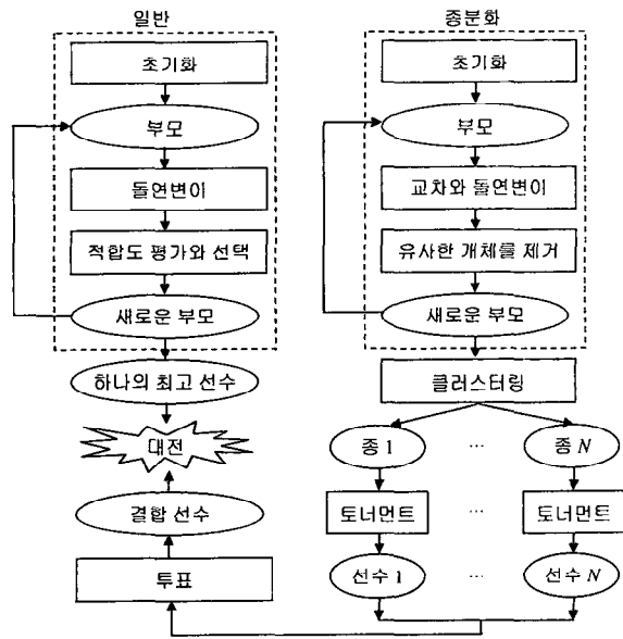
그림 7. 전체 흐름도
