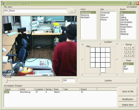
그림 3. 어노테이션 툴
