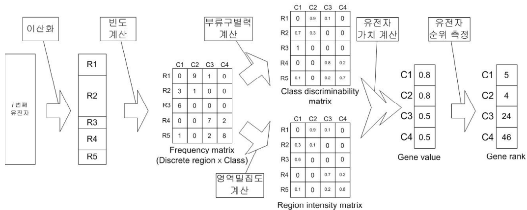
그림 1. 제안하는 유전자 선택 방법
